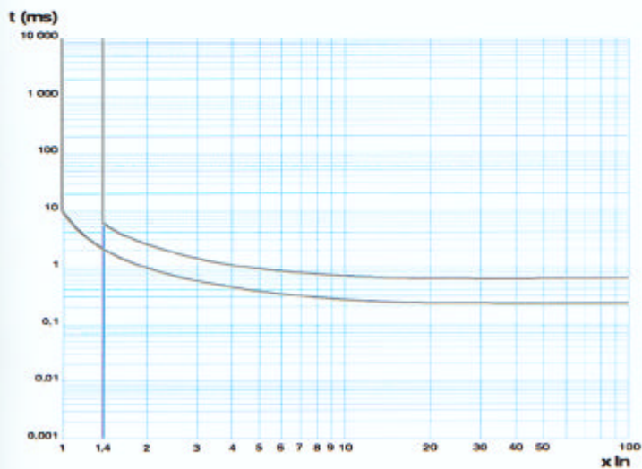
Série / Range 7000 Magnétiques purs / Magnetics only
