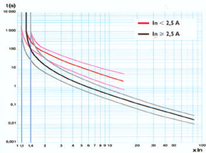
Série / Range 7000 Thermiques 2 à 20 A / Thermals 2 to 20 A
