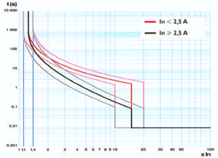
Série / Range 7000 Magnéto-thermiques courbe D / Thermal-magnetics curve D
