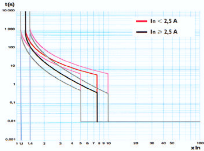
Série / Range 7000 Magnéto-thermiques courbe C / Thermal-magnetics curve C
