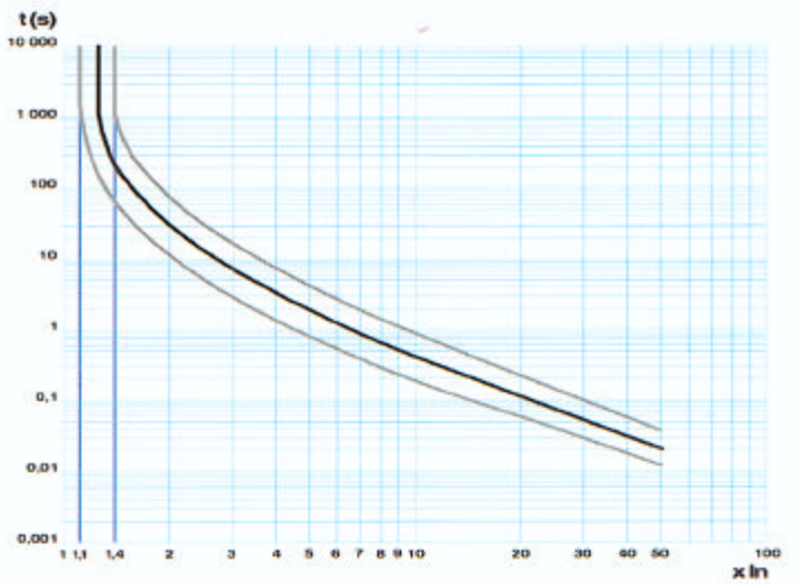
Série / Range 7000 Thermiques 21 à 40 A / Thermals 21 to 40 A
