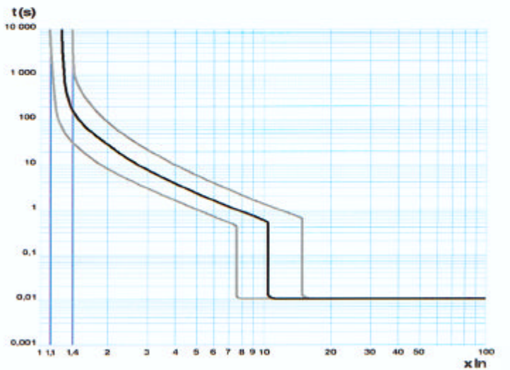
Série / Range 7500 Magnéto-thermiques 2 à 70 A / Thermal-magnetics 2 to 70 A
